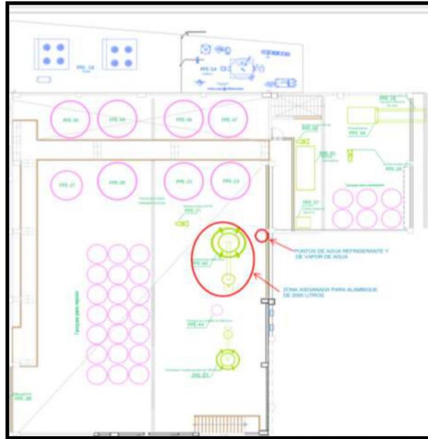
Anexo 01: Nave principal de la planta piloto, de color rojo los puntos asignados para la instalación del alambique de 2000 litros de capacidad y los puntos de agua y vapor requeridos para su instalación.
