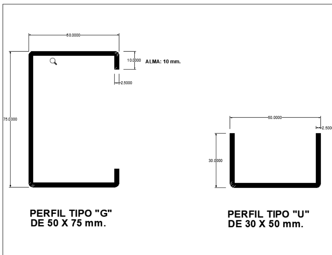
Figura N° 1 Perfil de Estructura
